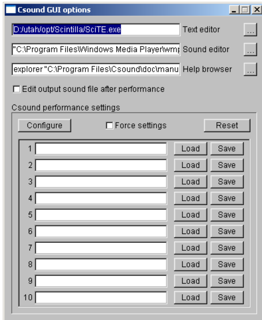
Figure 2.10.: Configuring csound5gui
