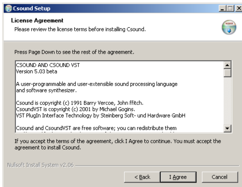
Figure 2.3.: Csound License
