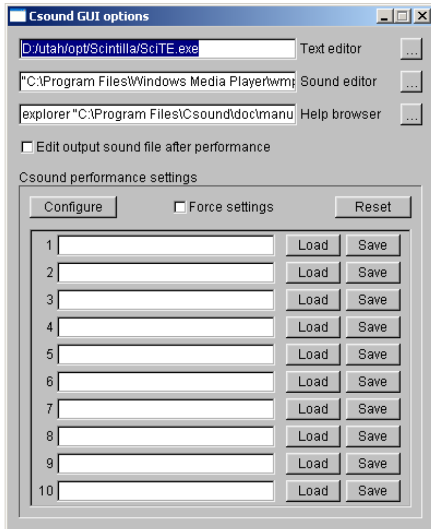
Figure 2.10.: Configuring csound5gui
